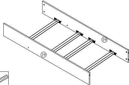
19-ALT KARYOLA SAĞ SOL TRAVERS
