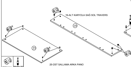
19-ALT KARYOLA SAĞ SOL TRAVERS
